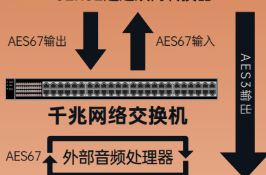
AE-6703 AES67/AES3 32x32通道双向转换器
