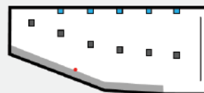
Vistas laterales que muestran las opciones para el altavoz de pared lateral en cines que no utilizan altavoces de techo
