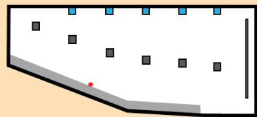
Виды сбоку, с вариантами боковых динамиков для кинозалов с потолочными динамиками
